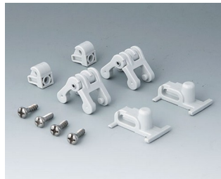
C7100142 Inside hinge PC
